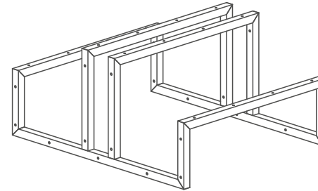
ESTRUCTURA SOPORTE: Tubos \square 40 mm. Acero al carbono galvanizado
